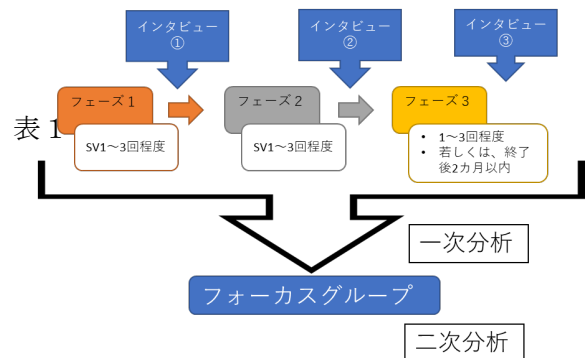
図1:研究の流れ
